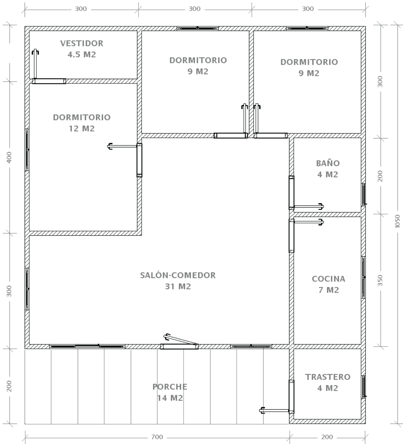
MODELO FRAN 80.5 M 2 + 14M 2 PORCHE
